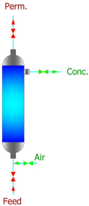
3.7 Air Scourge
