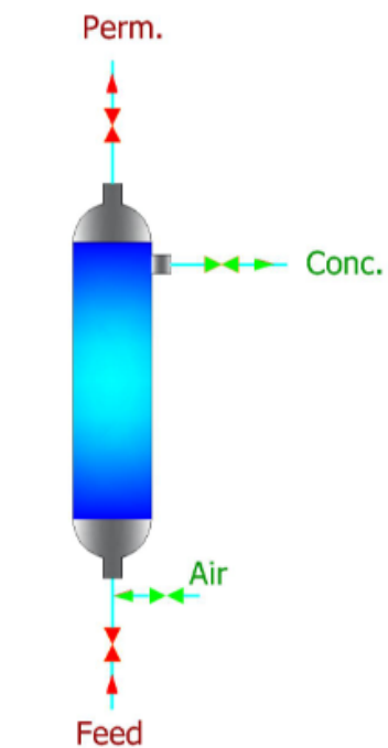
3.2 Air Scourge
