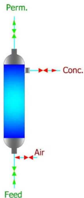
1.2 Filtration
