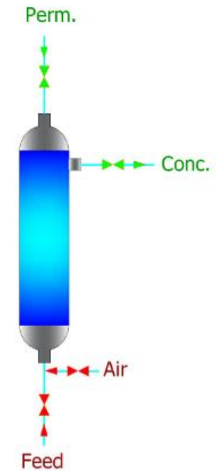
2.4 BW Top
