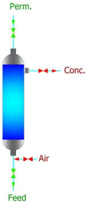
2.3 BW Bottom
