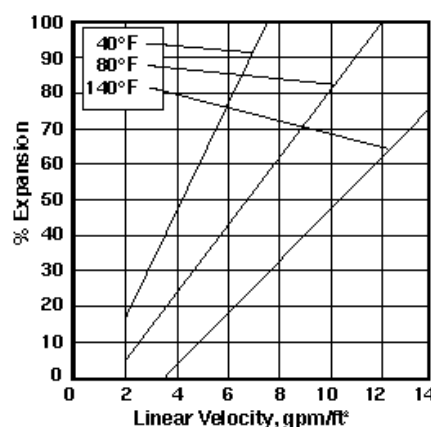
Fig. 2 : Bed Expansion
