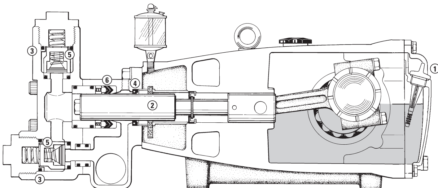
Models 6771, 6775, 6777
