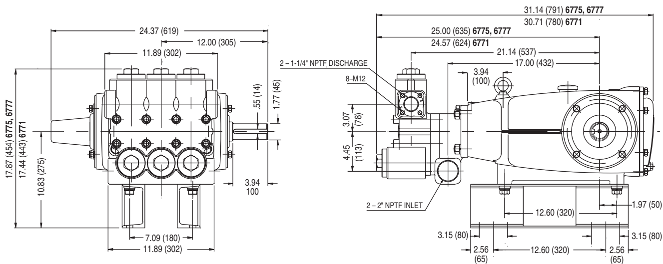
Models 6771, 6775, 6777
