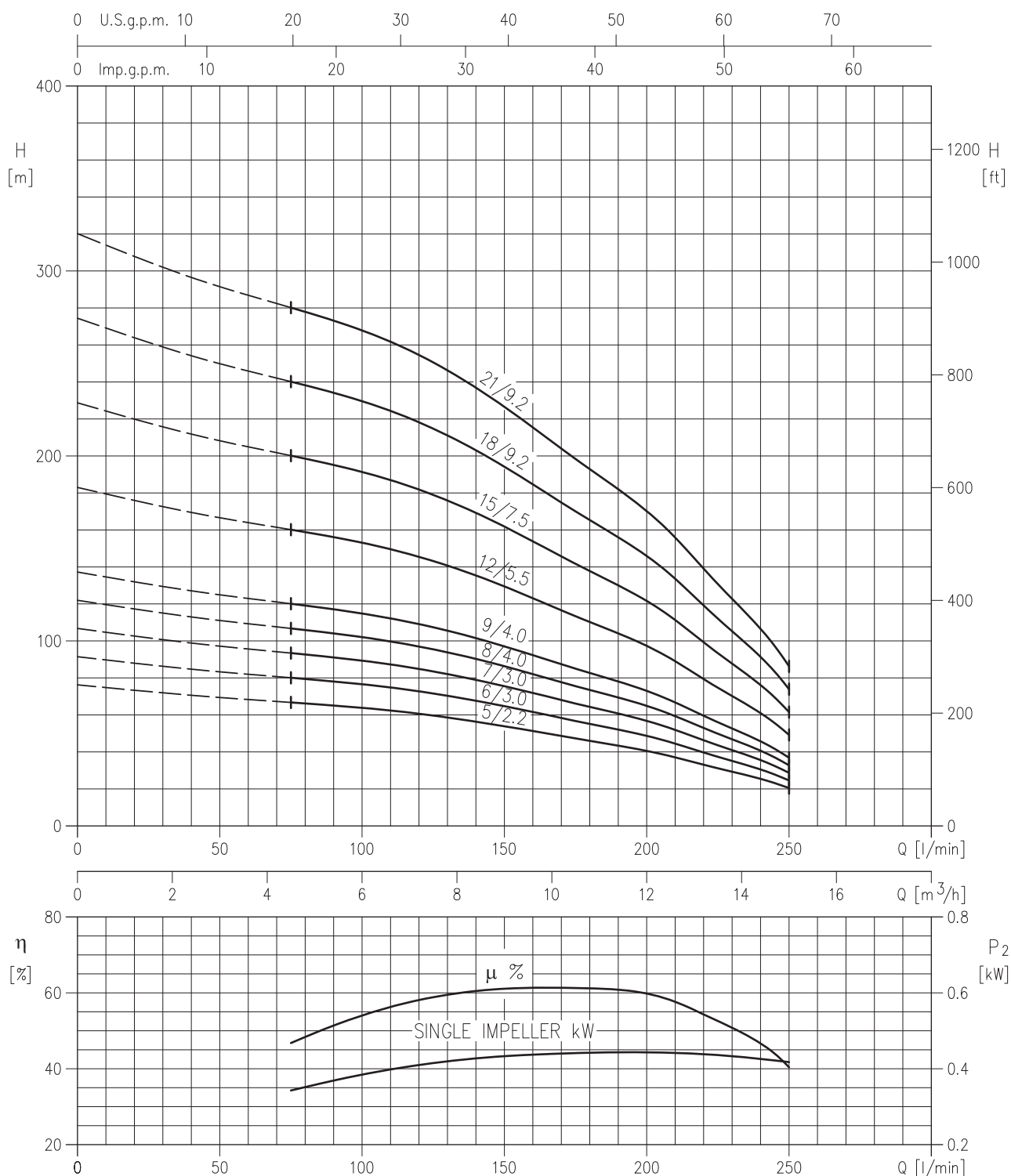
SF6 R10 MEI > 0.60 - Impeller diameter = 118 mm
