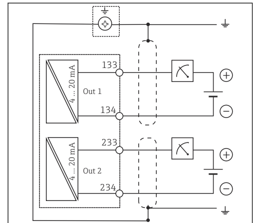
15 Wiring diagram
