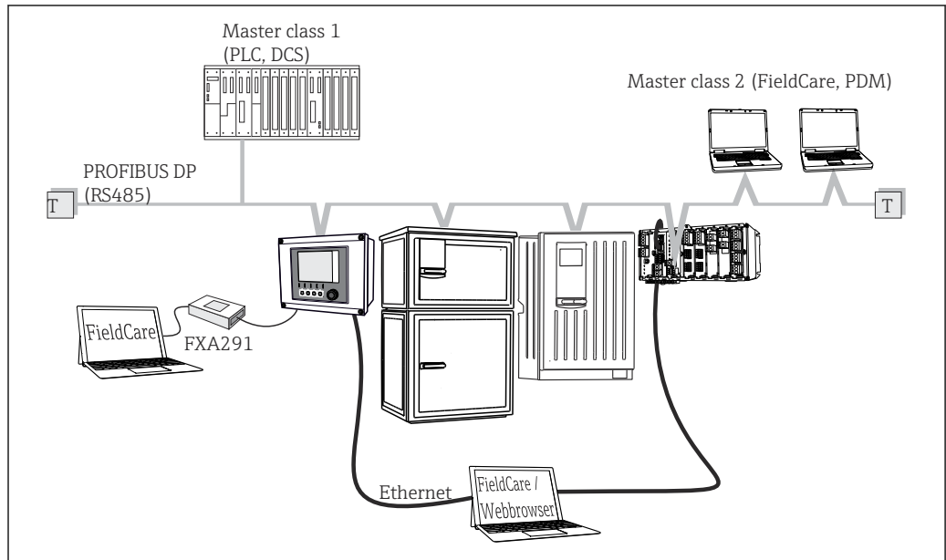
22 PROFIBUS DP
