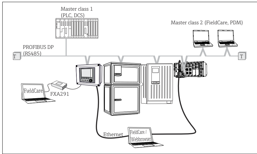
32 PROFIBUS DP
