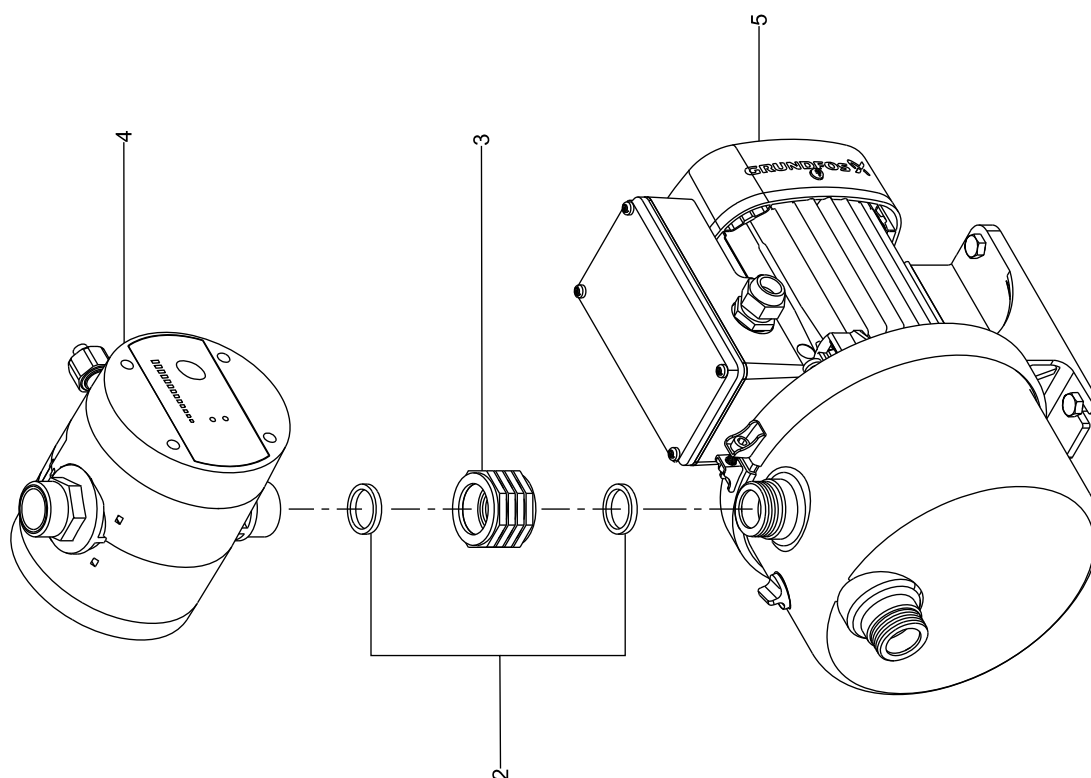
JP Booster PM 1 / PM 2
