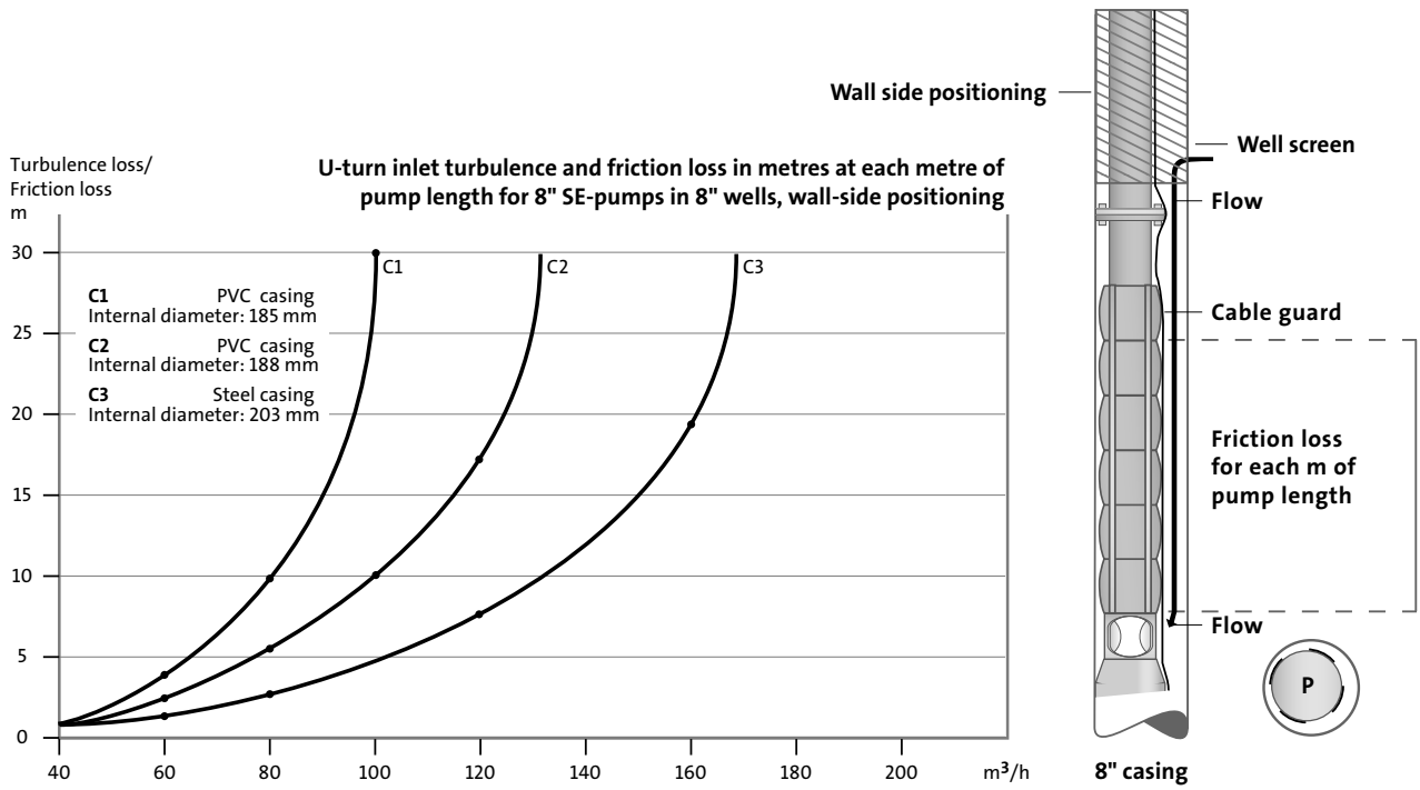
Fig. 55 U-turn, 8"
