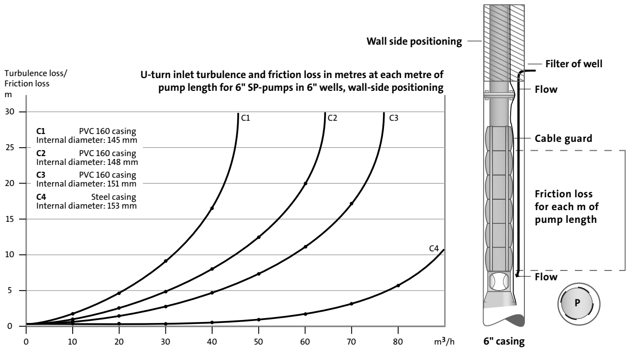
Fig. 54 U-turn, 6"
