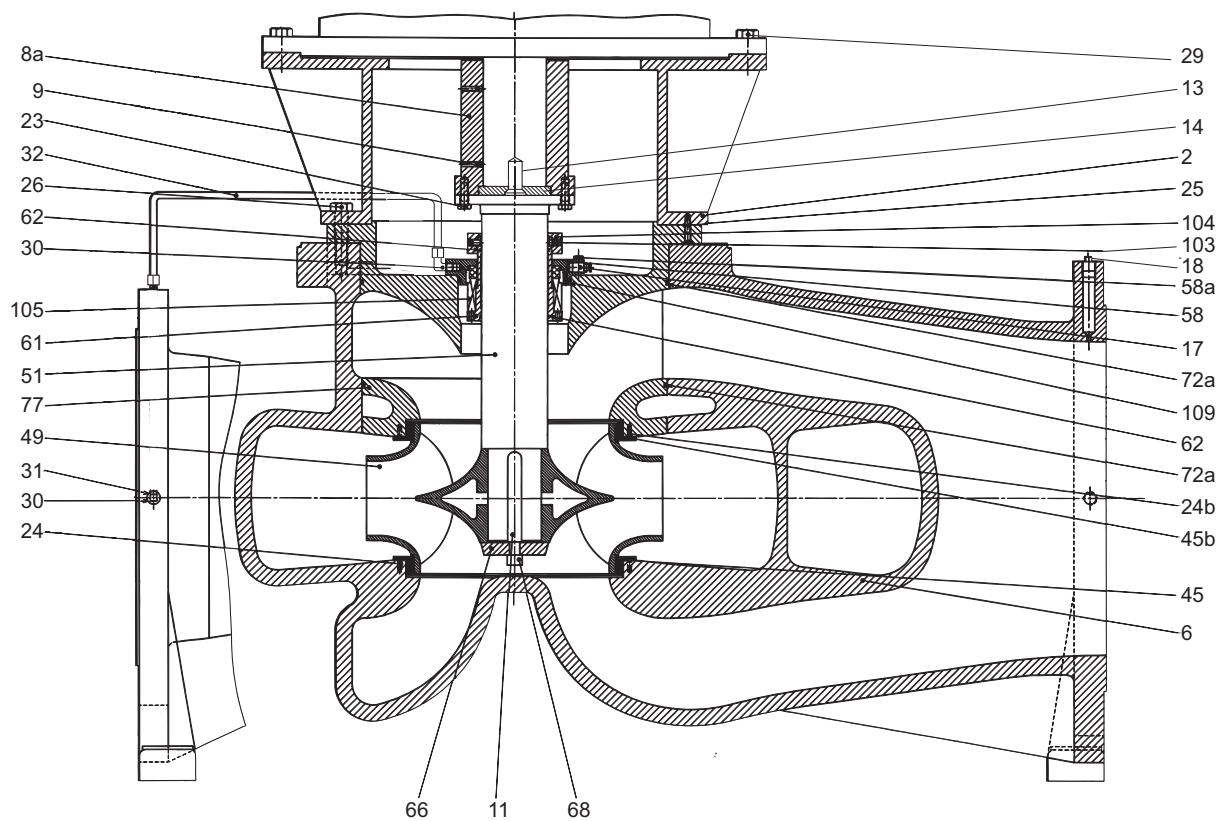
TP 400, 25 bar
