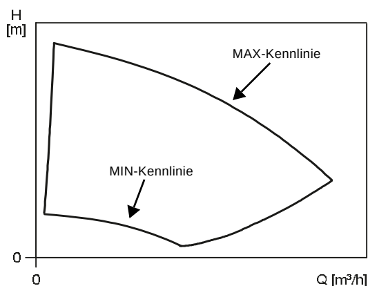
Abb. 20 MIN- und MAX-Kennlinie
