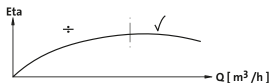
Abb. 26 Optimaler Betriebspunkt
