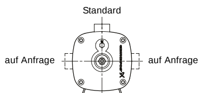
Abb. 45 Mögliche Anordnung des Druckstutzens
