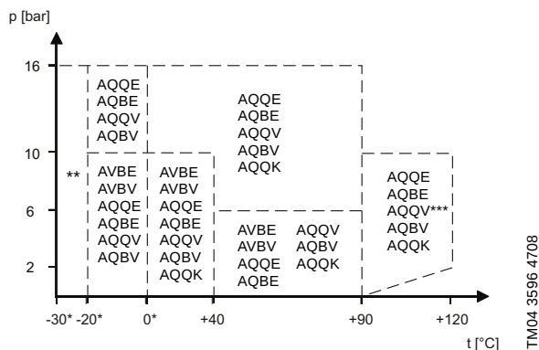
Abb. 12 Diagramm zur Auswahl der Gleitringdichtung
