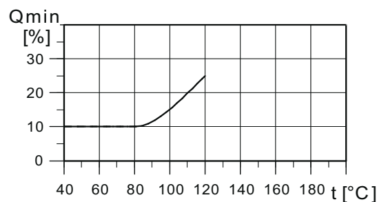
Abb. 31 Mindestförderstrom
