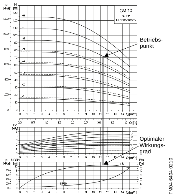
Abb. 27 Beispiel für den Betriebspunkt einer CM-Pumpe
