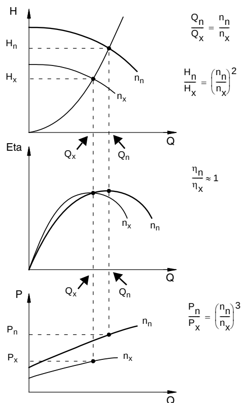
Abb. 21 Affinitätsgleichungen
