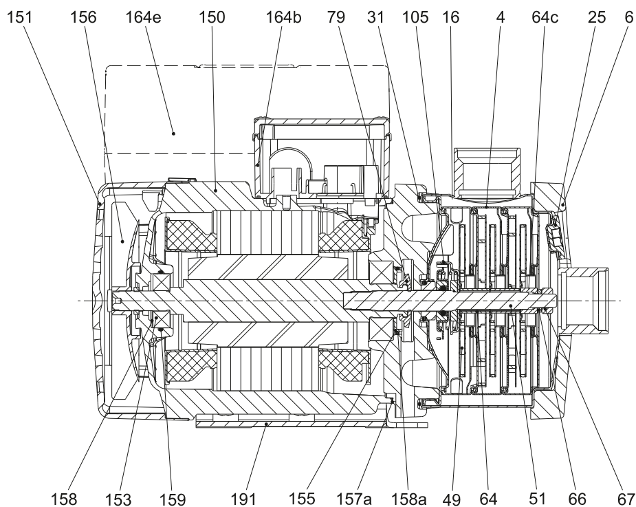
Abb. 17 CM(E) 1-3 mit Motor MG(E) 71
