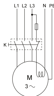
Abb. 39 Drehstrommotor mit einer Heizeinheit zur Vermeidung von Kondensation
