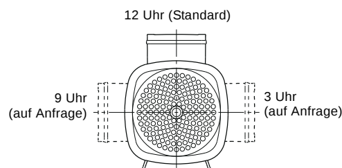
Abb. 44 Mögliche Klemmenkastenstellungen bei den Motorbaugrößen 71 und 80
