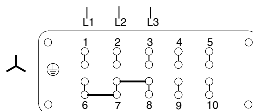
Abb. 35 Steckeranschluss für Stern-Schaltung
