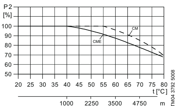
Abb. 9 Zusammenhang zwischen der Motorausgangsleistung ( P_2 ) und der Umgebungstemperatur/Aufstellungshöhe
