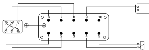
Abb. 34 Steckeranschluss am Motor
