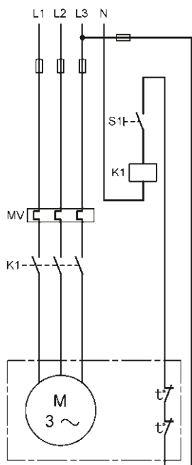
Abb. 43 Drehstrommotor mit Thermoschaltern
