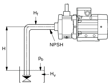
Abb. 13 Mindestzulaufdruck, NPSH
