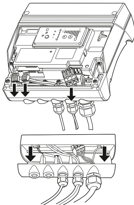
Abb. 37 Anordnung der abnehmbaren Kabeleinführungsleiste
