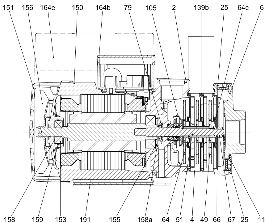
Abb. 16 CM(E) 1-3 mit Motor MG(E) 71
