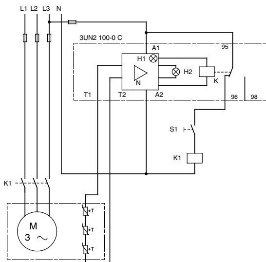
Abb. 41 Drehstrommotor mit PTC-Fühlern
