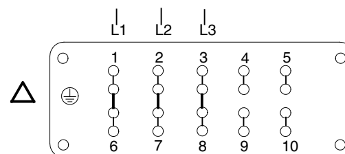
Abb. 36 Steckeranschluss für Dreieck-Schaltung
