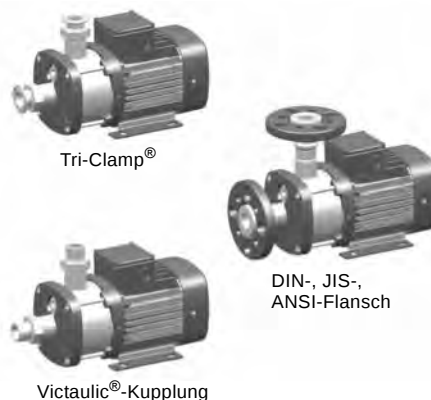
Abb. 28 Beispiele für Pumpenanschlüsse
