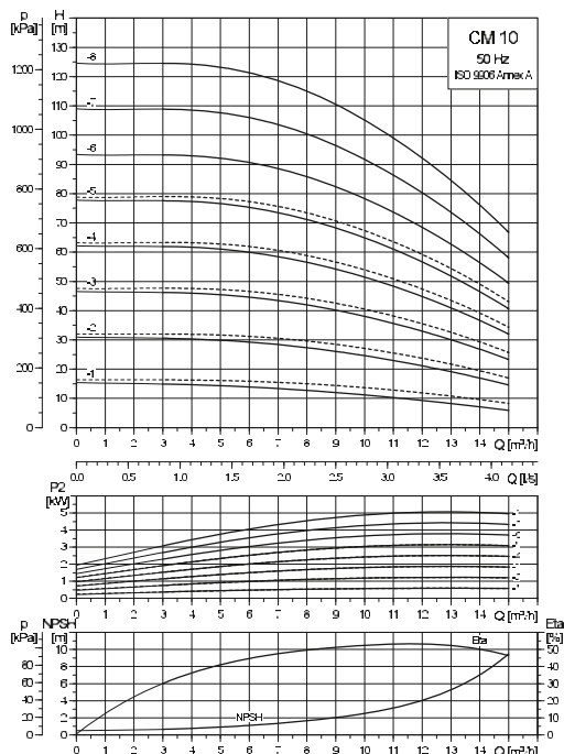
Abb. 24 Beispiel für ein Kennliniendiagramm
