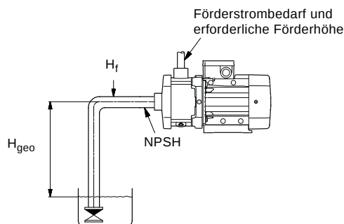
Abb. 25 Auslegungsdaten
