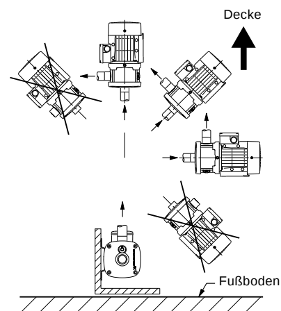
Abb. 10 Pumpenanordnungen
