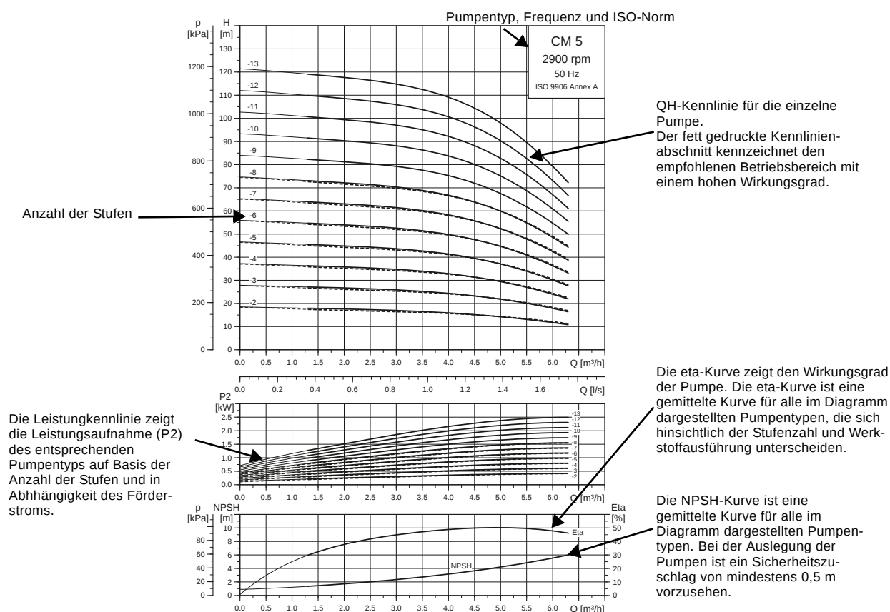
Abb. 30 Lesen der Kennlinien
