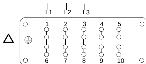
Abb. 16 Steckeranschluss für Dreieck-Schaltung
