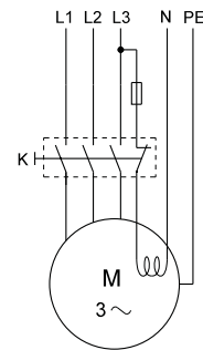
Abb. 19 Drehstrommotor mit Heizeinheit zur Vermeidung von Kondensation
