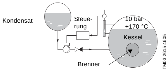
Abb. 3 Kesselspeisung mit drehzahlgeregelten Pumpen
