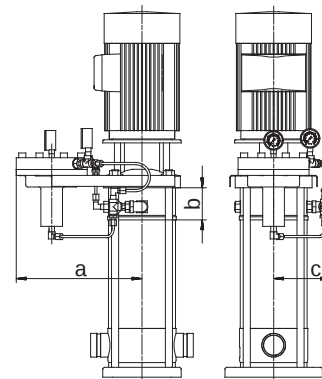
Abb. 34 Maßskizze
