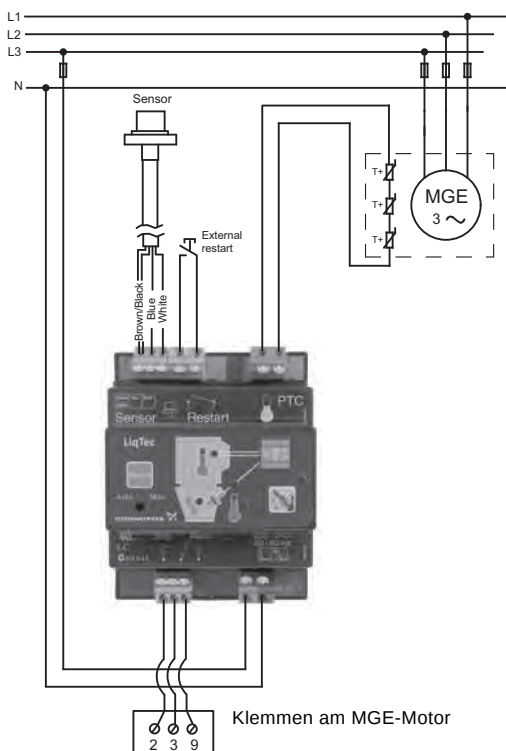
Abb. 62 LiqTec angeschlossen an einen MGE-Motor
