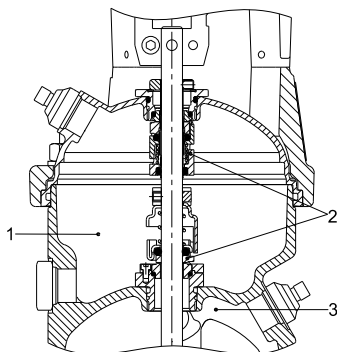
Abb. 26 CR 1s bis 5 mit Back-to-Back-Dichtungsanordnung
