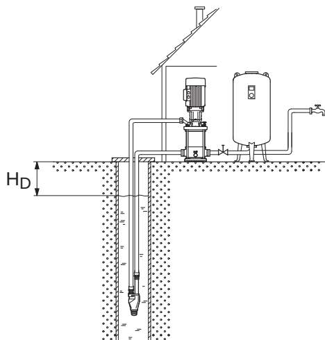
Abb. 57 Anlage mit CR(I)-Tiefsaugepumpe
