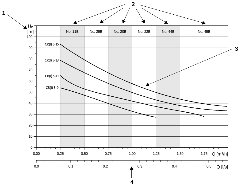
Abb. 84 Beispiel für die Kennlinie einer CR-Tiefsaugpumpe
