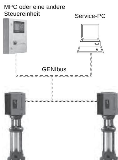
Abb. 79 Interne Buskommunikation
