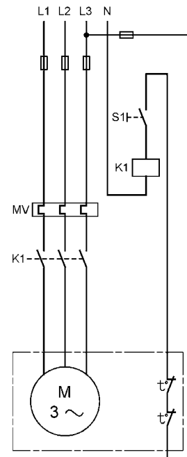
Abb. 23 Drehstrommotor mit Thermoschaltern
