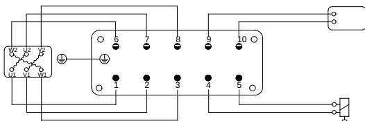
Abb. 14 Steckeranschluss vom Motor
