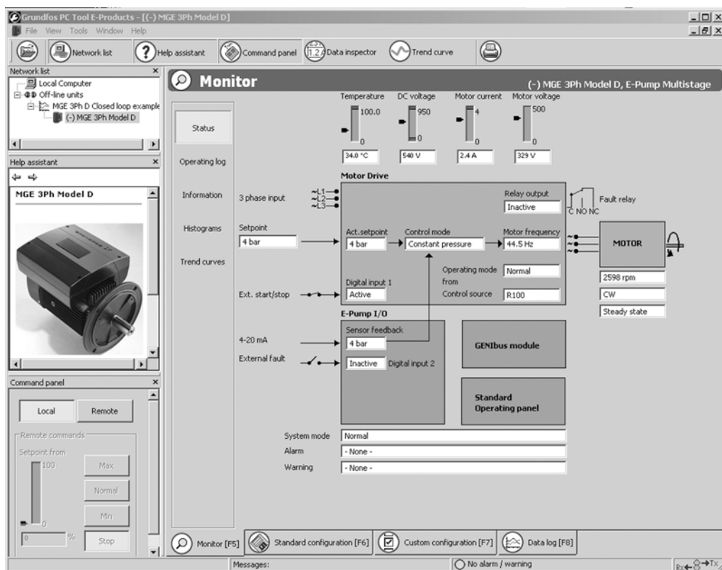
Abb. 83 Überwachungsfunktion
