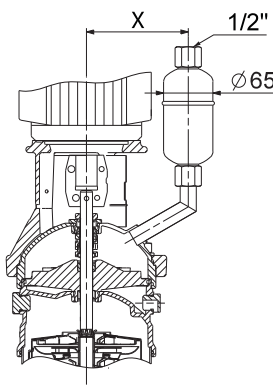
Abb. 47 Luftgekühlte Wellendichtungskammer
