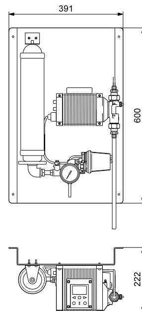
Abb. 31 Maßskizze
