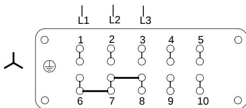
Abb. 15 Steckeranschluss für Stern-Schaltung
