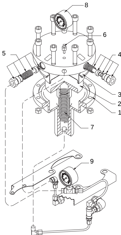
Abb. 33 Komponenten des Druckverstärkers
