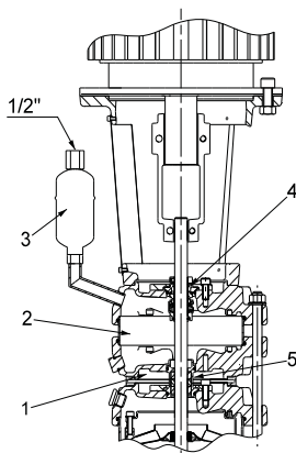
Abb. 44 CR 32, 45, 64 und 90 mit luftgekühlter Wellendichtungskammer
