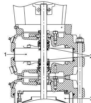
Abb. 28 CR 32 bis 90 mit Back-to-Back-Dichtungsanordnung
