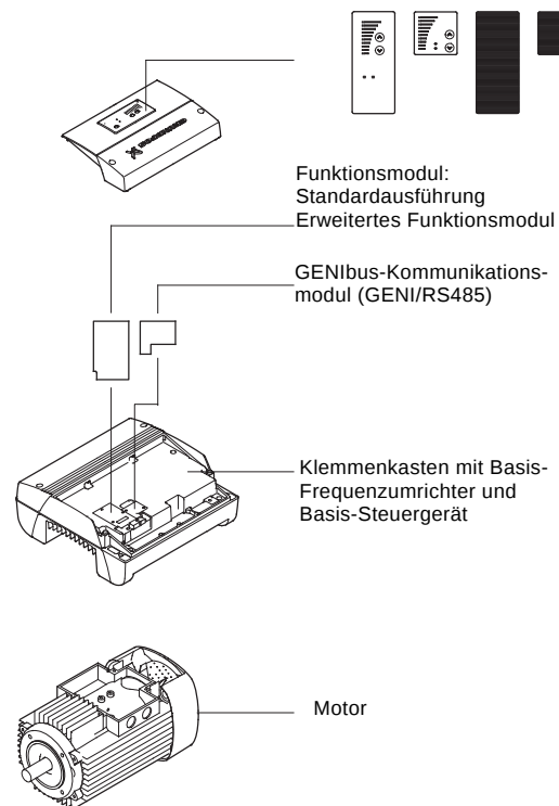
Abb. 75 Kombination der Motorkomponenten von kundenspezifisch hergestellten CRE-Pumpen
