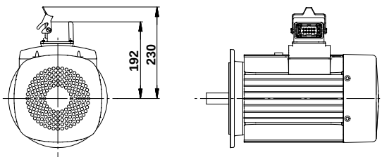
Abb. 13 Abmessungen 1,5 - 7,5 kW
