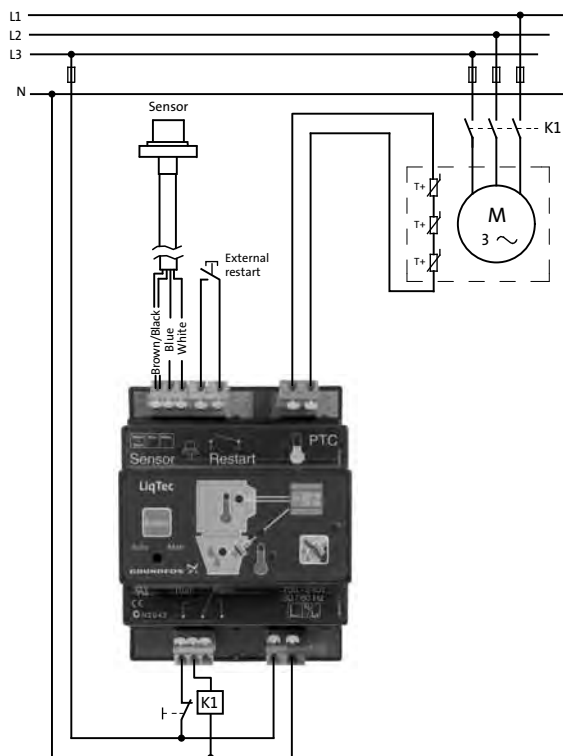
Abb. 61 LiqTec angeschlossen an einen ungeregelten Standardmotor
