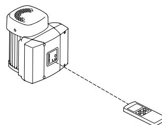
Abb. 77 Kommunikation der CRE-Pumpe mit der R100-Fernbedienung
