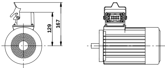
Abb. 12 Abmessungen 0,37 - 1,1 kW
