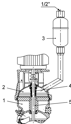
Abb. 42 CR 1s, 1, 3 und 5 mit luftgekühlter Wellendichtungskammer
