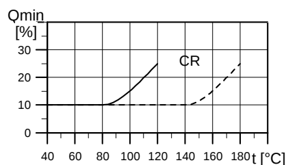
Abb. 86 Mindestförderstrom
