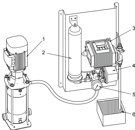
Abb. 30 CR-Pumpe mit Dosierpumpe
