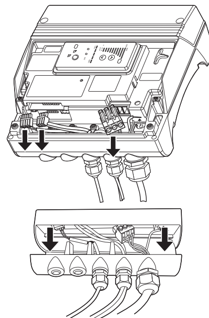
Abb. 17 Anordnung der abnehmbaren Kabeleinführungsleiste am Klemmenkasten des Motors und der Stecker für den Netzanschluss, den Sensor und die Datenübertragung
