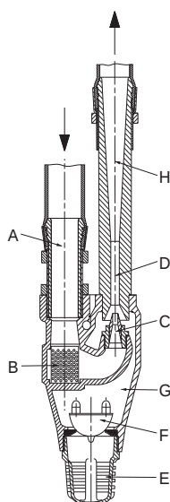
Abb. 58 Schnittzeichnung vom Ejektor
