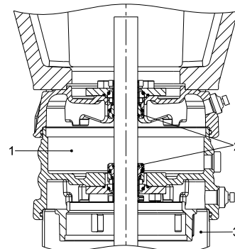
Abb. 29 CR 120 bis 150 mit Back-to-Back-Dichtungsanordnung
