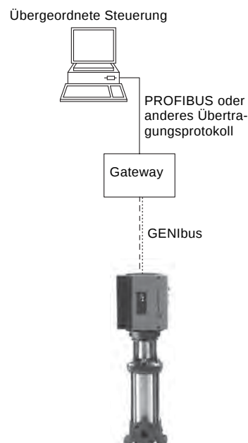
Abb. 80 Externe Buskommunikation
