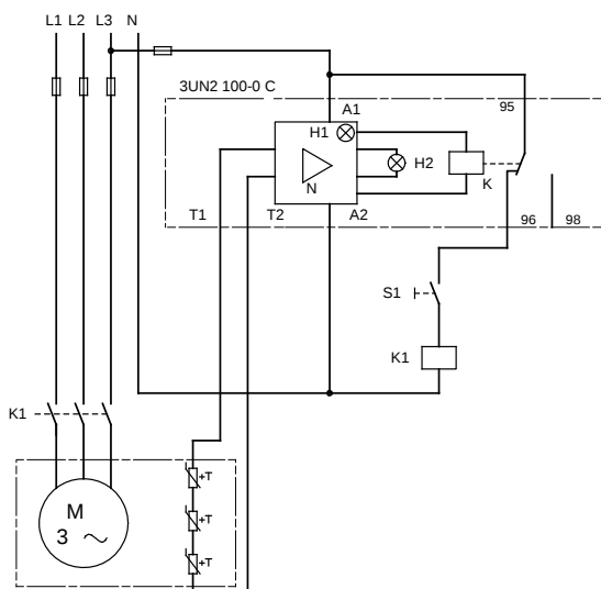
Abb. 21 Drehstrommotor mit PTC-Sensoren
