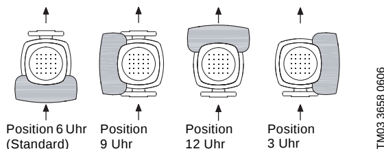
Abb. 24 Mögliche Anordnungen des Klemmenkastens
