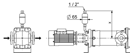
Abb. 48 Position der Entlüftungsvorrichtung bei horizontal aufgestellten CR-Pumpen in Hochtemperatursausführung
