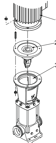
Abb. 59 Pumpe mit Lagerflansch
