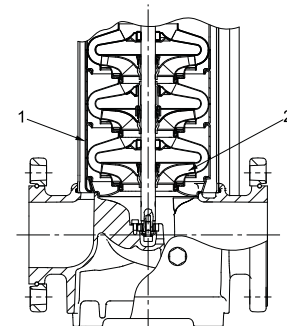
Abb. 54 Schnittzeichnung einer CR-Pumpe mit niedrigem NPSH-Wert
