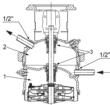
Abb. 35 CR 1s bis 20 mit Tandem-Dichtungsanordnung
