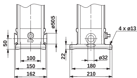
Abb. 63 TriClamp-Kupplung für CRI, CRN 1s, 1, 3 und 5
