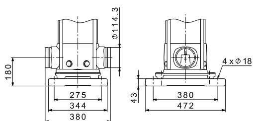
Abb. 71 PJE-Kupplung für CRN 120 und 150
