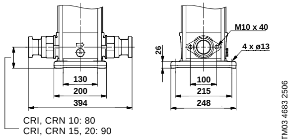
Abb. 66 Anschluss nach EN/DIN 11851 für CRI, CRN 10, 15 und 20
