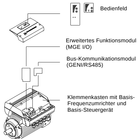
Abb. 73 Hardwarekombination einer CRE-Standardpumpe
