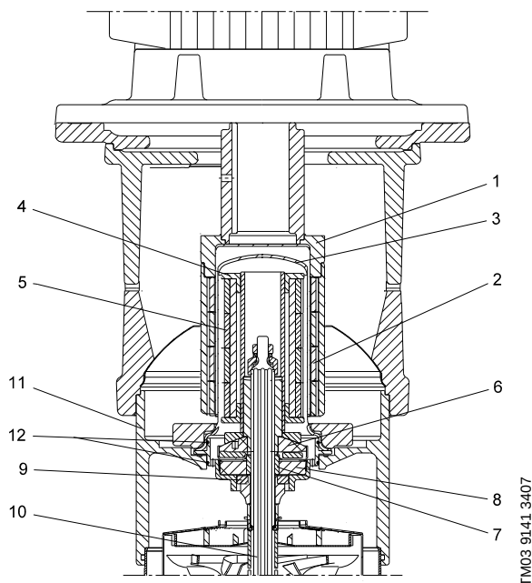
Abb. 51 Schnittzeichnung der Magnetkupplung MAGdrive
