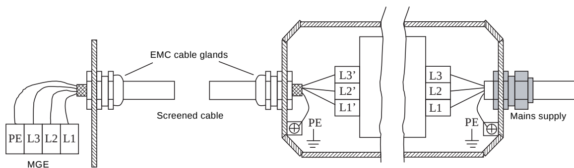
Fig. 145 Wiring diagram
