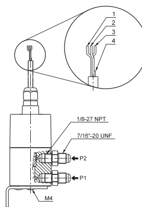
Fig. 136 Wiring
