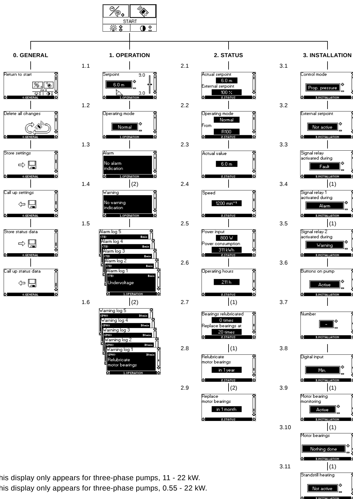
Fig. 78 Menu overview
