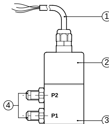
Fig. 134 DPI sensor
