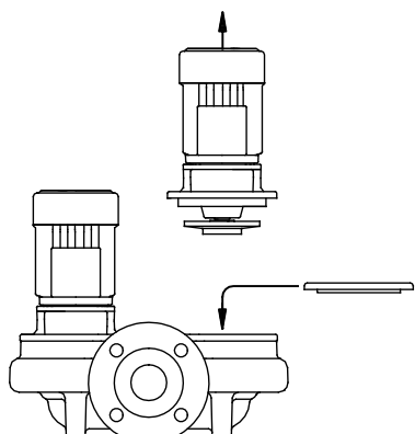
Fig. 112 Blanking flange
