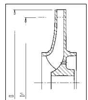
Reduzierung des Laufrad-Außendurchmessers für Kreiselpumpe mittels Drehen.
