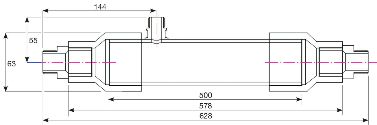
Figure 2: ZW700B-250 Dimensions
