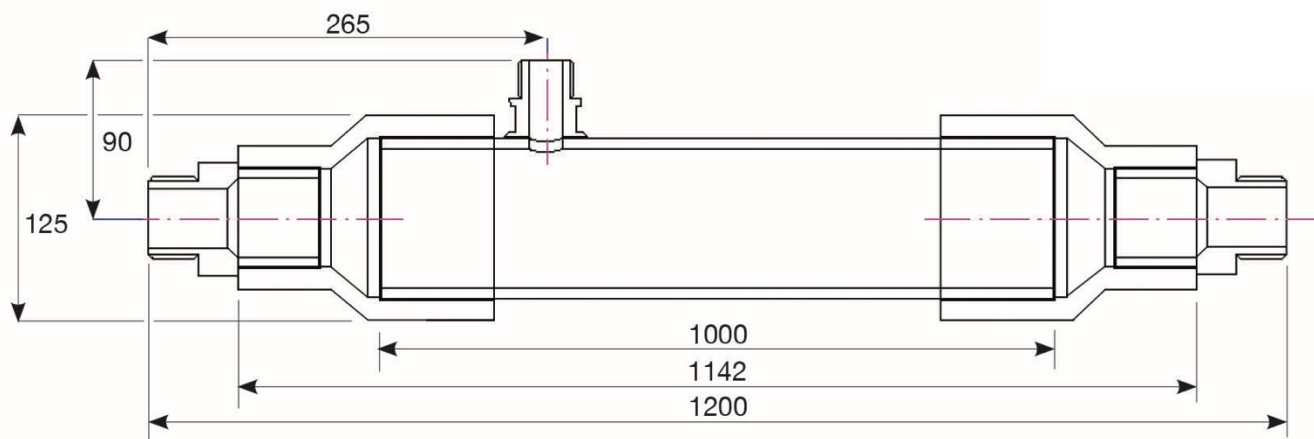
Figure 2: ZW700B-4100 Dimensions
