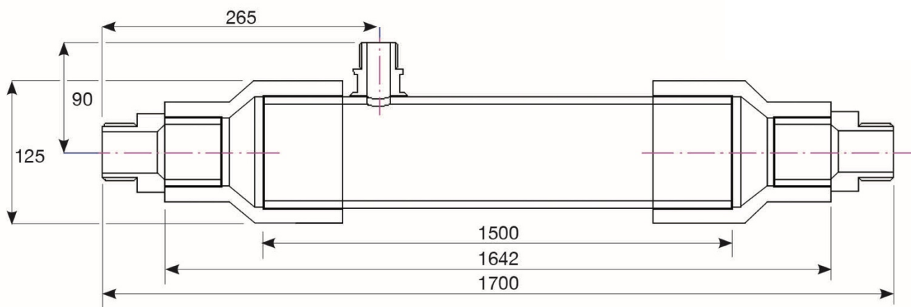
Figure 2: ZW700B-4150 Dimensions
