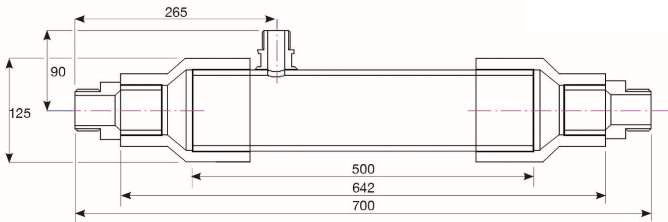
Figure 2: ZW700B-450 Dimensions
