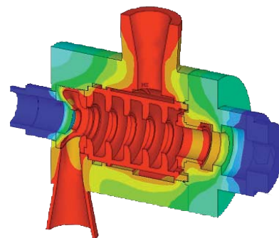
Análise computadorizada para otimizar a distribuição de temperaturas em várias condições
