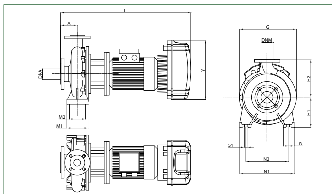
NKM-GE 40-250/260
