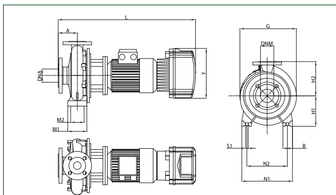
NKM-GE 40-200/219
