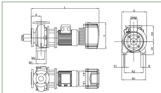
NKM-GE 50-125/141 - NKM-GE 50-160/177
