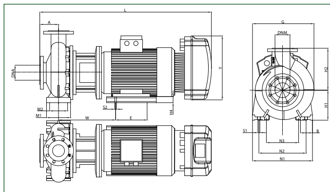
NKM-GE 100-200/214
