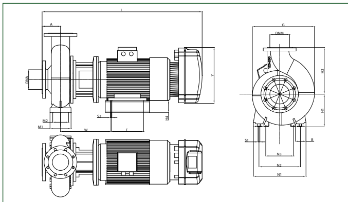
NKM-GE 125-250/243 - NKM-GE 150-200/218
