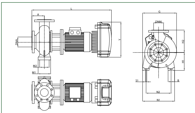
NKM-GE 100-200/200
