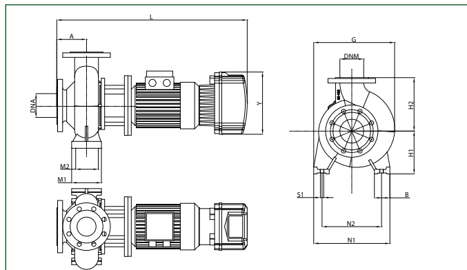
NKM-GE 80-250/270 - NKM-GE 80-315/305
