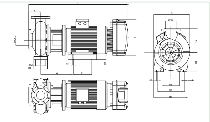
NKM-GE 100-250/250 - NKM-GE 100-250/270
