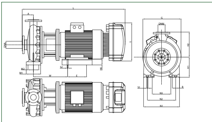
NKM-GE 80-160/177 - NKM-GE 80-200/222
