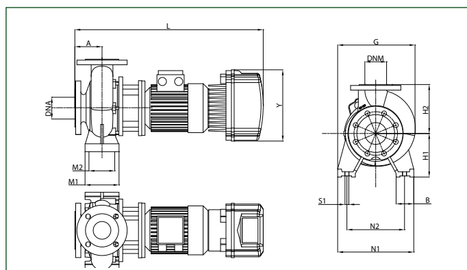
NKM-GE 65-125/144 - NKM-GE 65-160/153
