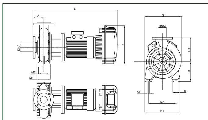
NKM-GE 65-200/210
