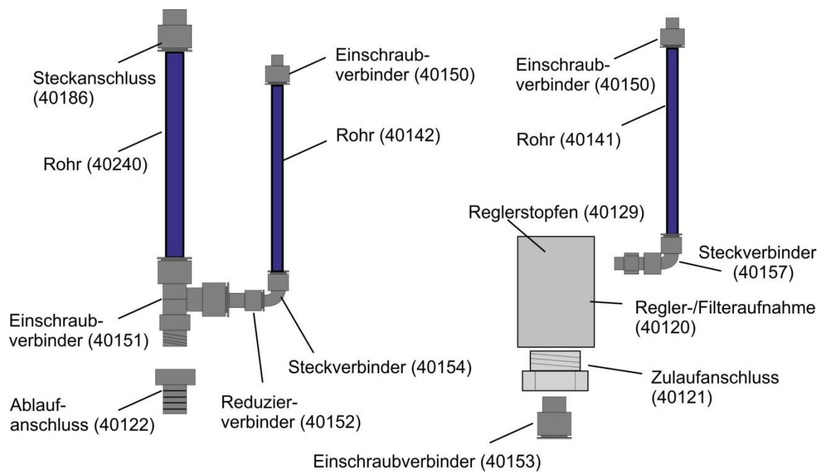
Innere Verbindungsteile Testomat 2000® / ECO, Verrohrung
