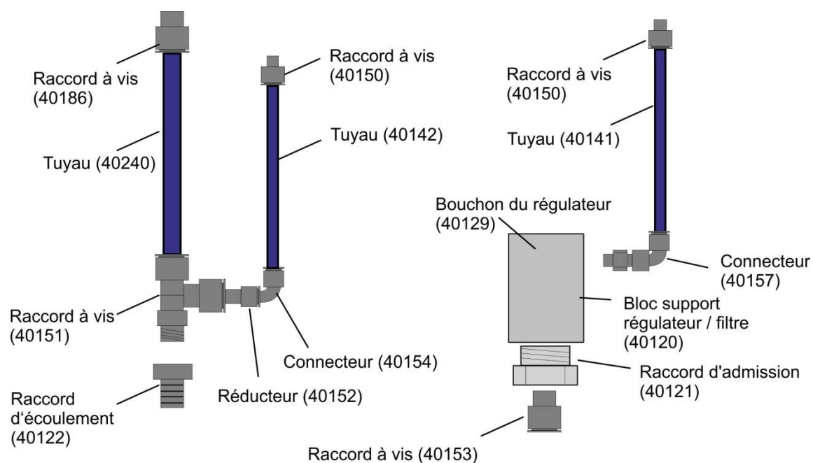
Parties intérieures de la connexion pour Testomat 2000® / ECO, Montage des tuyaux
