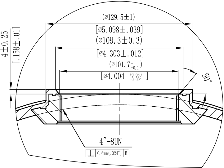
Part A 1:2
