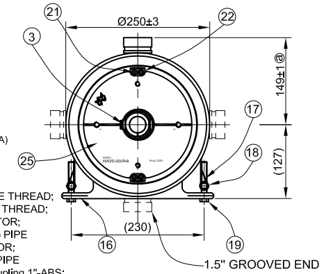
II DETAIL 1:1
