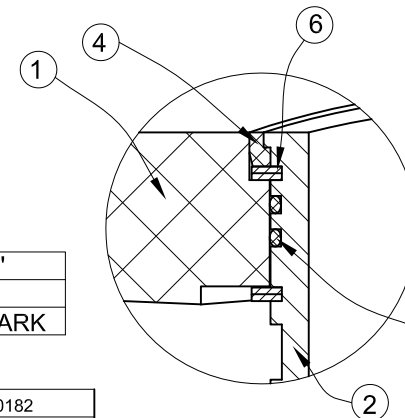
I DETAIL 1:1
