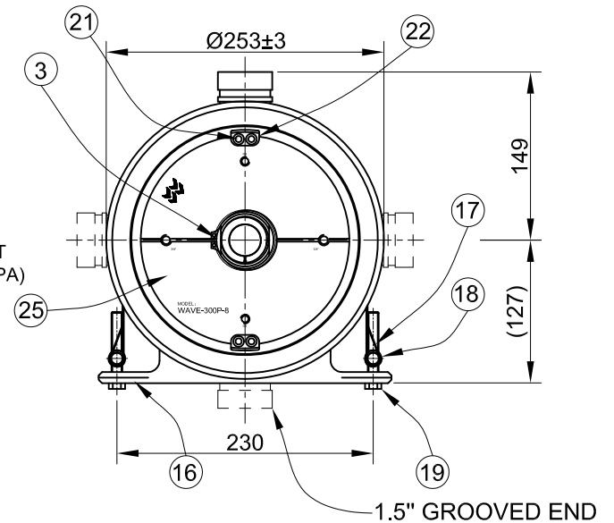
II DETAIL 1:1
